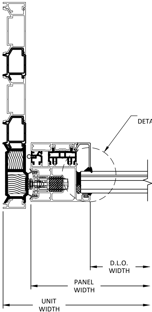
E 18 HORIZONTAL SECTION ALS-C JAMB 3 TRACK
