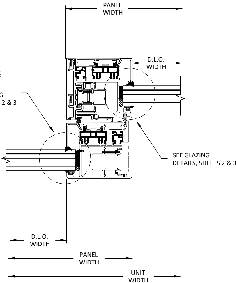
G 18 HORIZONTAL SECTION ALS-C INTERLOCK
