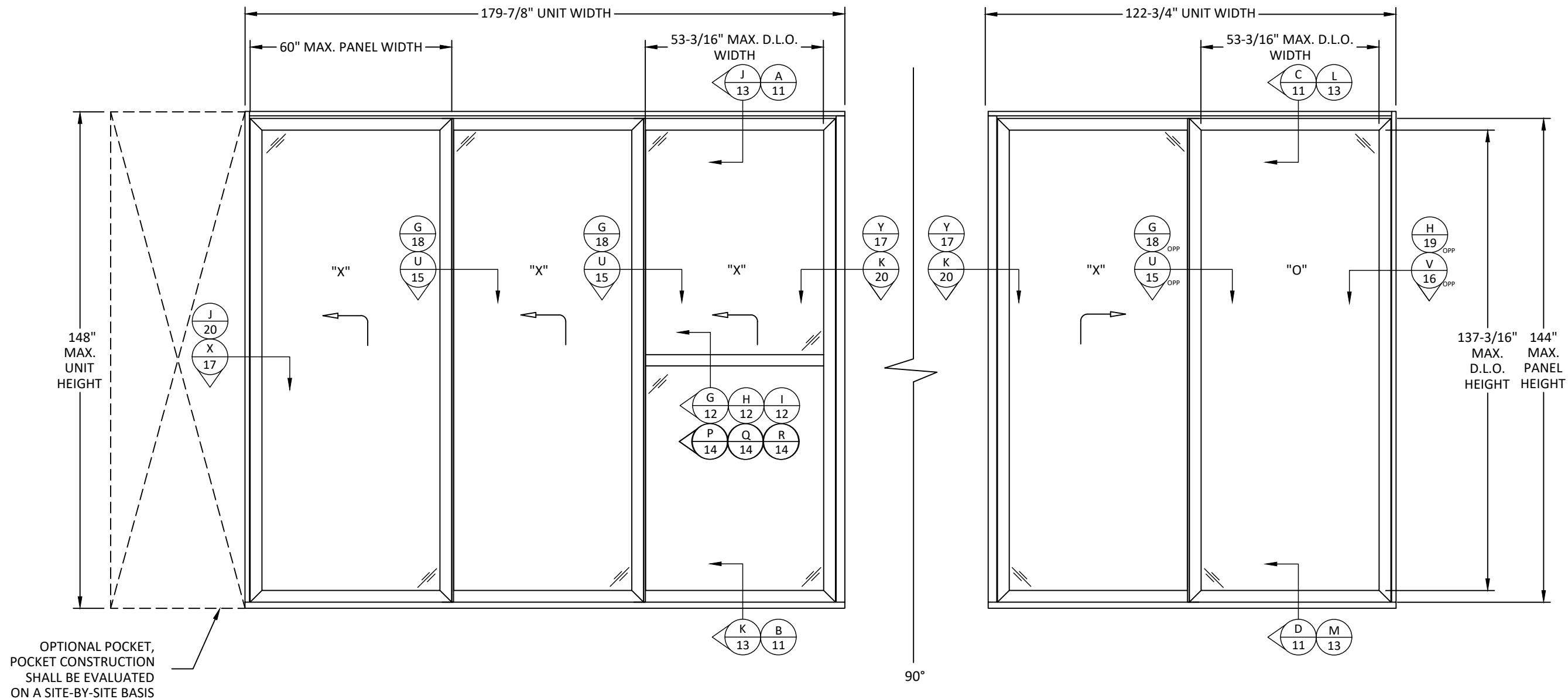
ELEVATION 90° CORNER PXXX-XO
